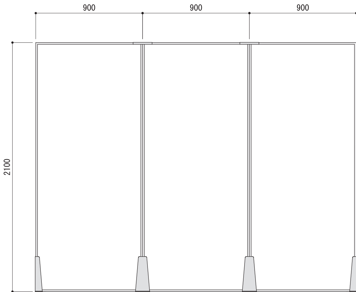
立面図
